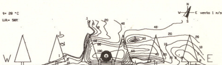
Figura 9 schiera del piano quotato della copertura percentuale riferita alla distribuzione ottenuta con l'atomizzatore tradizionale C a 1500 \text{ dm}^3/\text{ha} .
