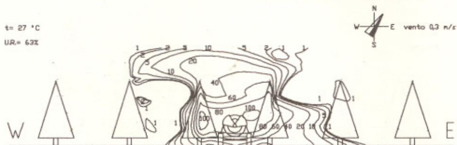
Figura 10 distribuzione delle gocce, visualizzata con le curve di isocopertura, relativa all'irroratrice senovente a polverizzazione mista B operante a 1500 \text{dm}^3/\text{ha} .
