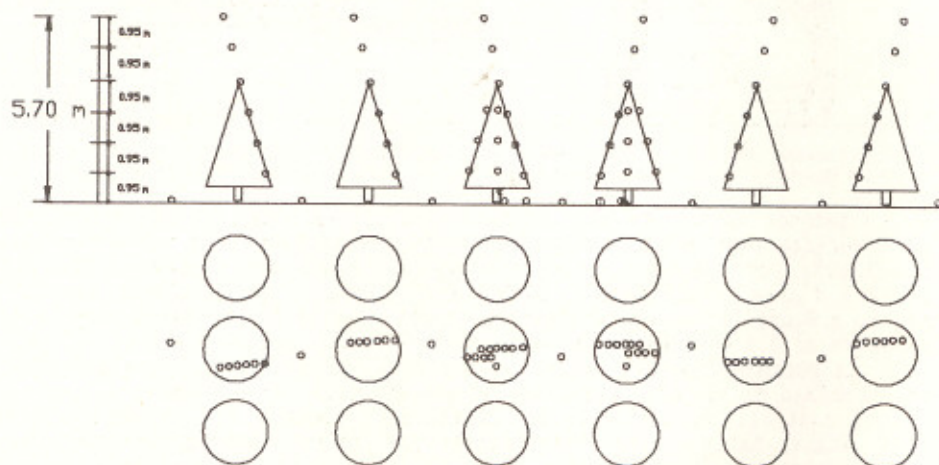
Figura 2 - Prospetto (in sito) della distribuzione spaziale delle carte idrosensibili utilizzate per rilevare la distribuzione delle gocce. Le stesse carte sono visibili in pianta anche nello schema in basso, dove si evidenzia in particolare la dislocazione sfalsata per evitare la rutila interferenza nella captazione delle gocce.
