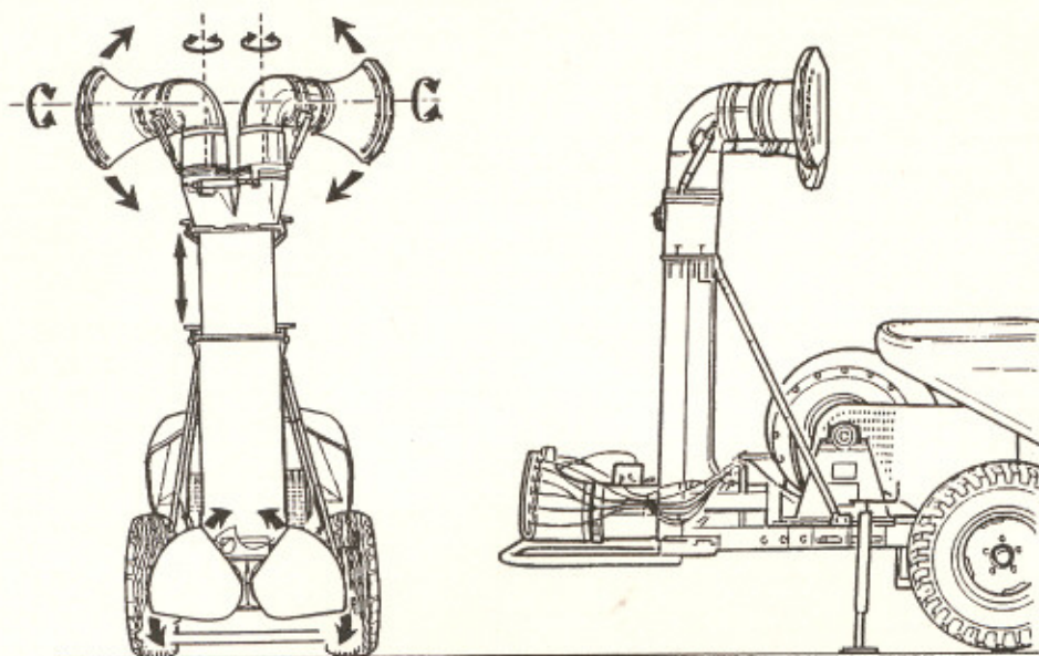
Figura 1: l'irroratrice A a polverizzazione pneumatica con getto mirato e carica elettrostatica operante a basso volume. Nello schema di sinistra sono indicate, con frecce, le possibili regolazioni dei quattro diffusori
